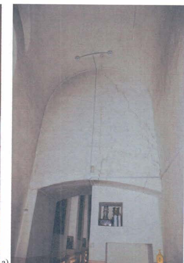
Фото 17. ОКН «Церковь святителя Николая Чудотворца». Фрагменты интерьера (а) южное крыло притвора, б) северное крыло притвора). Наличие трещин в штукатурном слое стен и сводов.
