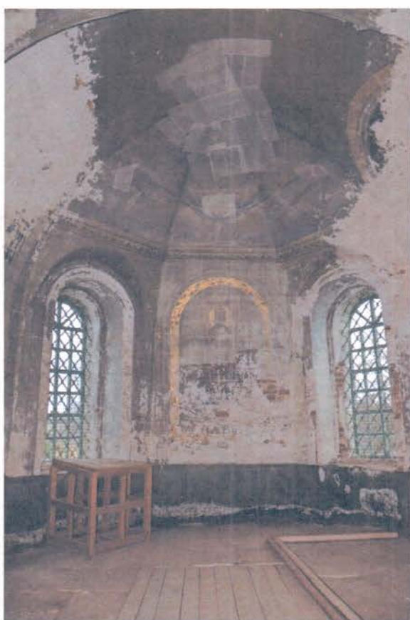
Фото 28. ОКН «Церковь святителя Николая Чудотворца». Фрагменты интерьера (апсида алтаря). Наличие трещин в летнем храме, на локальных участках фиксируется увлажнение и биопоражение (мох, плесень) нижней части стен, небольшие механические повреждения кладки алтаря, множественные трещины в штукатурном слое, утраты и отслоение штукатурного слоя.
