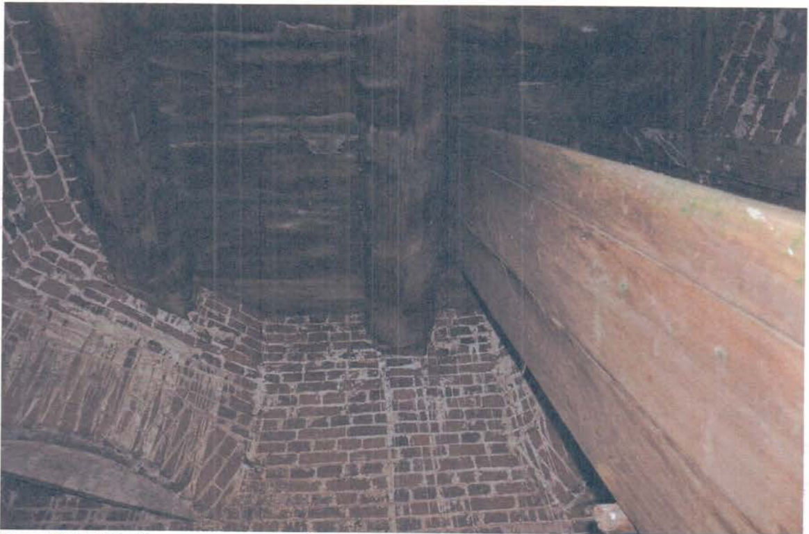
Фото 22. ОКН «Церковь святителя Николая Чудотворца». Фрагмент интерьера (колокольня). Наличие следов замачивание древесины перекрытий колокольни атмосферными осадками.
