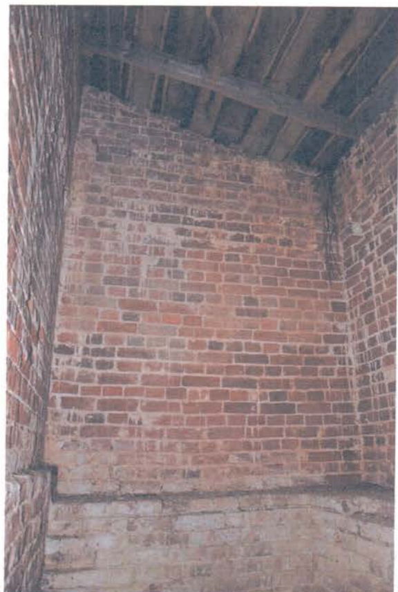
Фото 23. ОКН «Церковь святителя Николая Чудотворца». Фрагмент интерьера (колокольня). Удовлетворительное состояние конструкций крыши, лестницы на ярусы в удовлетворительном состоянии, загрязнение продуктами жизнедеятельности птиц.
