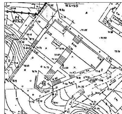
Генплан территории Сквера павшим героям
