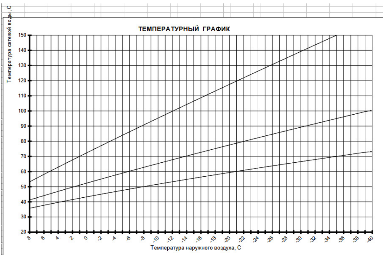
Рисунок 1.2.В – График зависимости температуры прямой и обратной сетевой воды от температуры наружного воздуха
